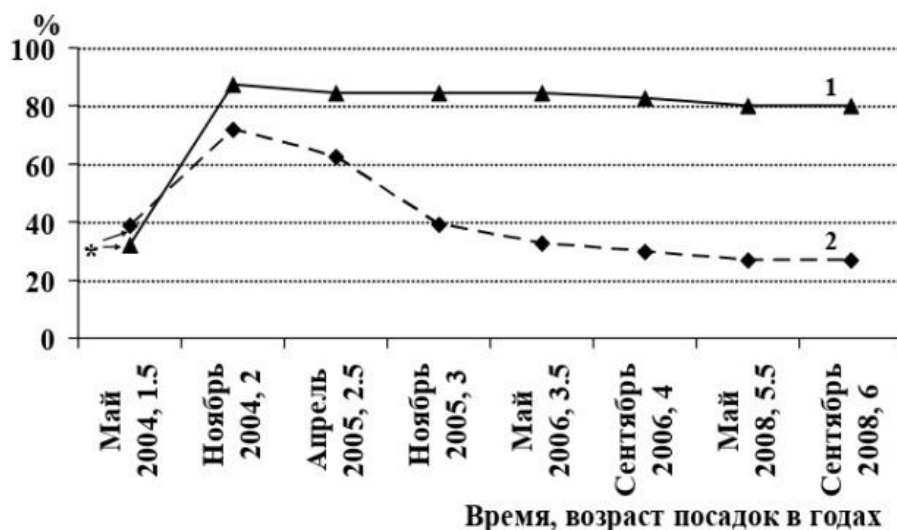
Рис. 24. Приживаемость (*) и сохранность (%) растений саксаула (а) и черкеза (б) в посадках на обсохшем дне Аральского моря 1) с поддерживающим поливом в первые два года и 2) в контроле – без полива (Кузьмина, Трешкин, 2010). Fig. 24. Survival (*) and adaptability (%) of Haloxylon aphyllum (а) and Salsola richteri (б) in automorphic solonchaks of the Aral Sea dried bottom 1) watered for the first 2 years and 2) not watered (Кузьмина, Трешкин, 2010).
