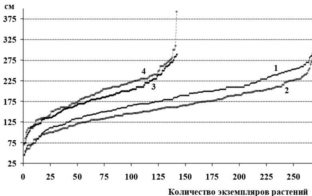
Рис. 26. Распределения высот (кривые 1 и 3) и диаметров крон (кривые 2 и 4) растений черного саксаула 6.5-летнего возраста (в мае 2009 г.) на грядковых посадках через 1 м (кривые 1 и 2) и через 2 м (кривые 3 и 4; Кузьмина, Трешкин, 2010). Fig. 26. Distribution of the height (curves 1 and 3) and crown diameter (curves 2 and 4) of the 6.5-year-old black saxaul in May 2009, planted on ridges every 1 m (curves 1 and 2) and 2 m (curves 3 and 4; Кузьмина, Трешкин, 2010).
