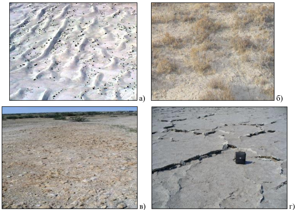
Фото 3. Лито-эдафические ландшафты Аральской впадины (Попов, 2017): а) песчаные, б) глинистые, в) солончаковые, г) каменистые. Photo 3. Litho-edaphic landscapes of the Aral basin (Попов, 2017): а) sandy, б) clay, в) saline, г) stony.
