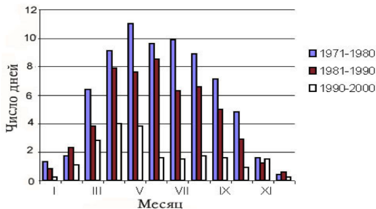
Рис. 9. Годовой ход повторяемости пыльных бурь в Муйнаке по десятилетиям (Чуб, 2007). Fig. 9. The annual frequency of dust storms in Muynak for decades (Чуб, 2007).
