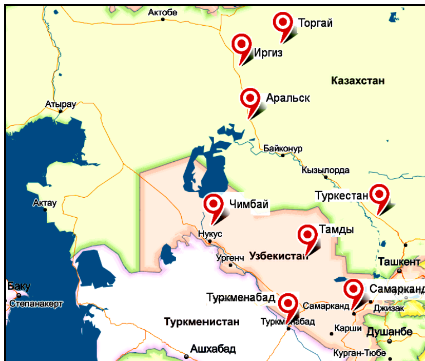
Рис. 3. Расположение метеостанций, входящих в состав Международной системы метеонаблюдений, в регионе Приаралья и сопредельных территориях Средней Азии, для которых был проведен анализ трендов основных метеорологических характеристик за многолетний период наблюдений (Кузьмина, Трешкин, 2016). Fig. 3. Location of weather stations that are part of the Worldwide Meteorological Observations System in the Aral Region and adjacent territories of Central Asia, for which the trend analysis of the main meteorological characteristics over a long period of monitoring was carried out (Кузьмина, Трешкин, 2016).
