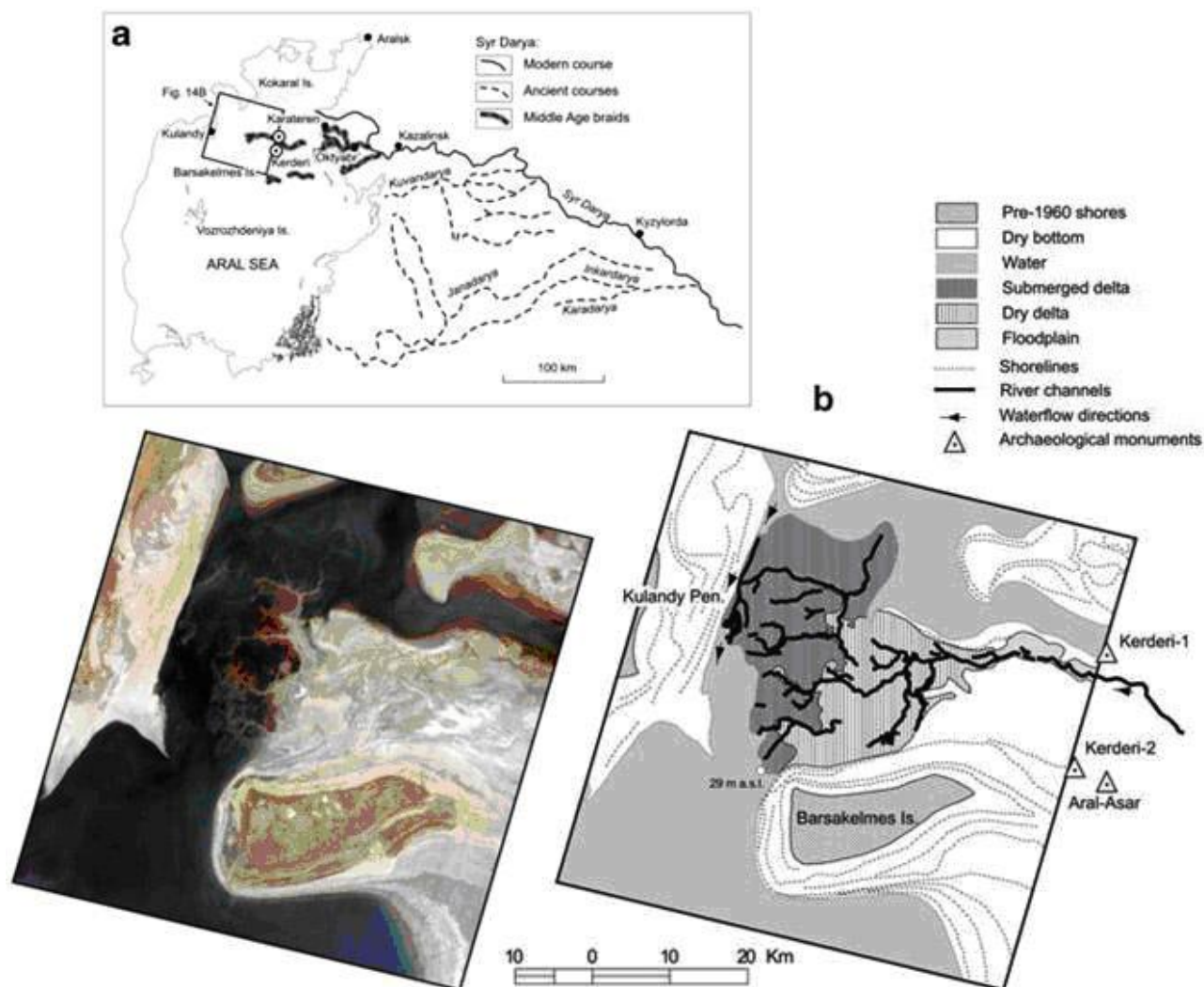
Рис. 18. Дельта Сырдарьи: а) основные русла и косы в Средние века, б) спутниковый снимок Астер 2004 года (слева) части дна Аральского моря между полуостровом Куланды и островом Барсакельмес и его интерпретация (справа) с протоками в средневековой дельте (Кривоногов, 2009). Fig. 18. The Syr Darya delta: a) its main courses and spits during the Middle Age, b) the ASTER satellite image of 2004 (left) showing a part of the Aral Sea bottom between the Kulandy Peninsula and Barsakelmes Island, and its interpretation (right) showing the delta during the Middle Age (Кривоногов, 2009).
