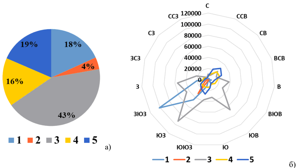
Рис. 11. Средний многолетний вынос массы песка 50% обеспеченности из очагов выветривания по рядам наблюдений метеостанций за 1966-1992 гг. на территории Казахстана, т/год: а) соотношение выноса из разных очагов, б) соотношение выноса песка по направлениям (создано по данным Семенов и др., 2006). Условные обозначения очагов солепылевыноса: 1 – о. Лазарева, 2 – о. Барса-Кельмес, 3 – Восточный, 4 – Сарышиганак, 5 – Кокаральский. Fig. 11. The average long-term removal of sand mass of 50% security from the centers of removal, according to observations on the weather stations for 1966-1992 in Kazakhstan,
