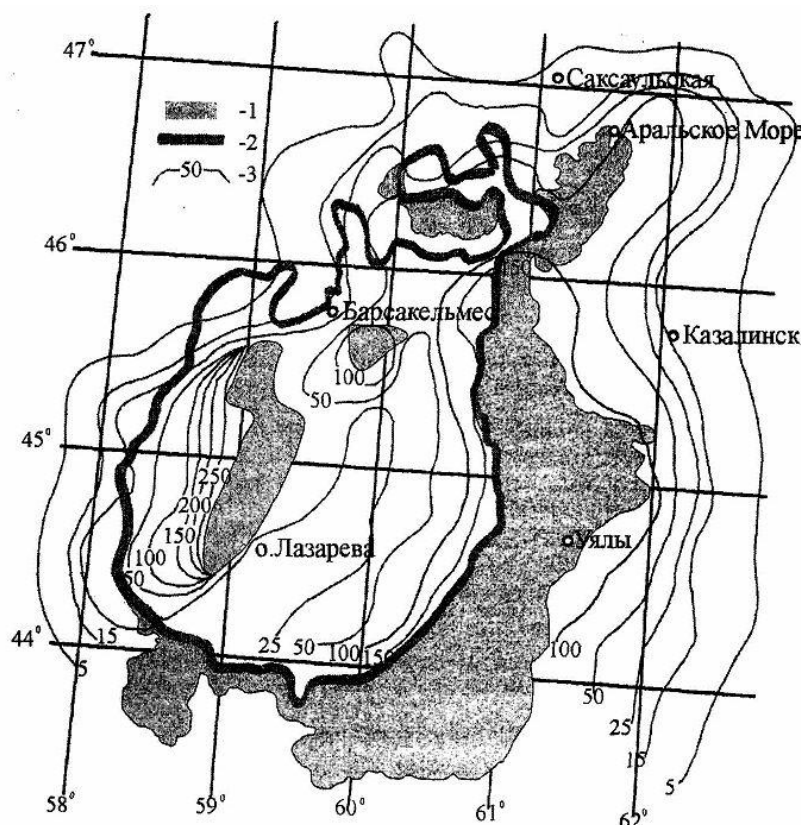
Рис. 12. Карта-схема средних многолетних значений сухих выпадений песчано-солевого аэрозоля ( t/km^2 в год) от дефляционных процессов на осушенной части дна Аральского моря. (Семенов и др., 2006). Условные обозначения: 1 – площадь осушенного дна моря, 2 – современная береговая линия, 3 – изолинии сухих выпадений. Fig. 12. Schematic map of the
