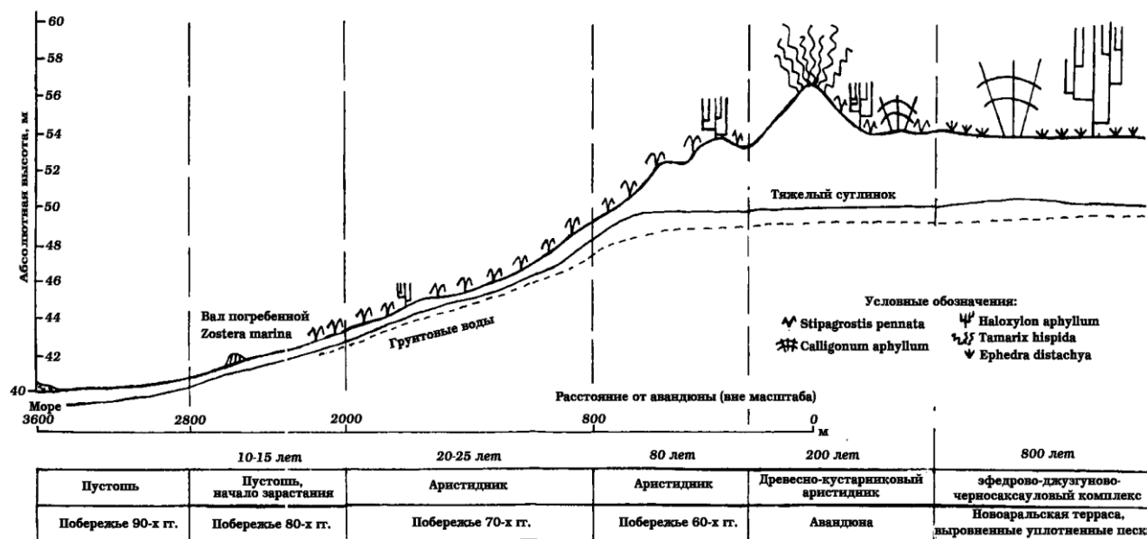
Рис. 21. Ключевые участки наблюдений за функциями растительности на трансекте песчаного побережья о. Барсакельмес (Панкратова, 2007). Fig. 21. Key sites where vegetation functions were observed on a transect of the sandy coast of the Barsakelmes Island (Панкратова, 2007).
