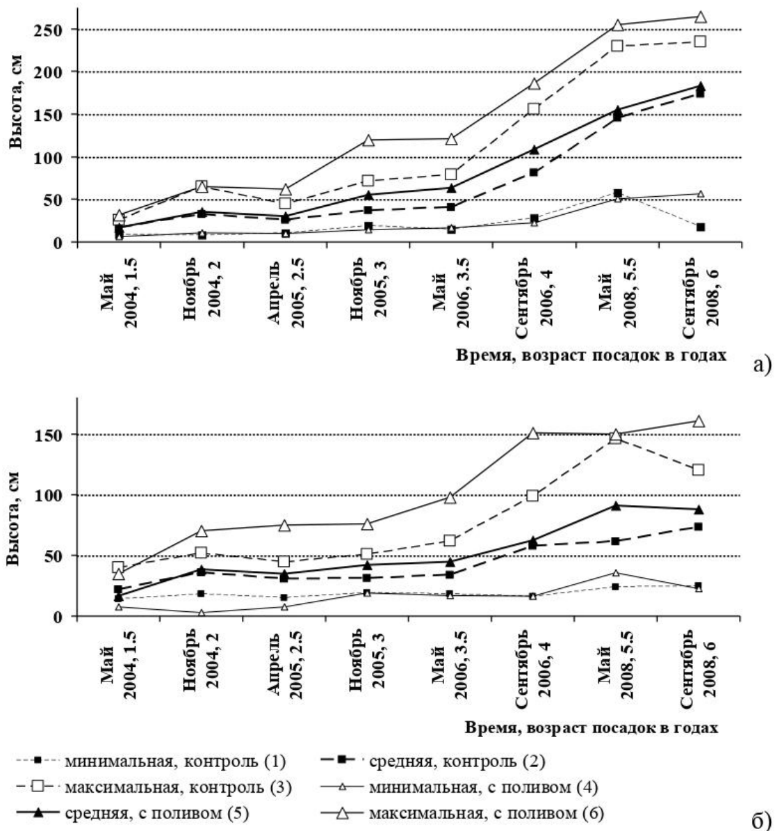
Рис. 25. Графики хода роста саксаула (а) и черкеза (б) с поддерживающим поливом в первые 2 года (сплошные кривые 4-6) и в контроле без полива (пунктирные кривые 1-3; Кузьмина, Трешкин, 2010). Fig. 25. The growth of Haloxylon aphyllum (а) and Salsola richteri (б) with sustaining watering during the first 2 years (curves 4-6) and without watering (dotted curves 1-3; Кузьмина, Трешкин, 2010).
