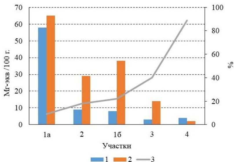
Рис. 22. Зависимость приживаемости саженцев саксаула от физико-химических свойств засоленных почв. Условные обозначения: 1 – суммарный эффект токсичных ионов, мг-экв/100 г почвы, 2 – содержание физической глины, %, 3 – приживаемость, % (Димеева, Пермитина, 2006). Fig. 22. Dependence of saxaul saplings survival rate on physical-chemical characteristics of saline soils. Notes: 1 – total effect of toxic ions, mg-eq/100 g of soil, 2 – content of clay, %, 3 – survival rate, % (Димеева, Пермитина, 2006).
